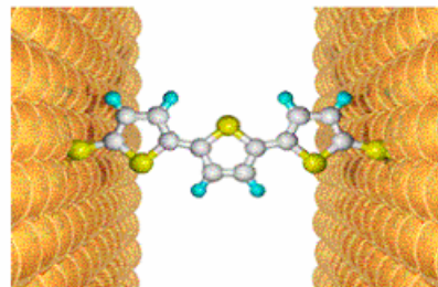
Représentation schématique d'une molécule de bithioterthiophène contactée par deux nanoélectrodes d'or
